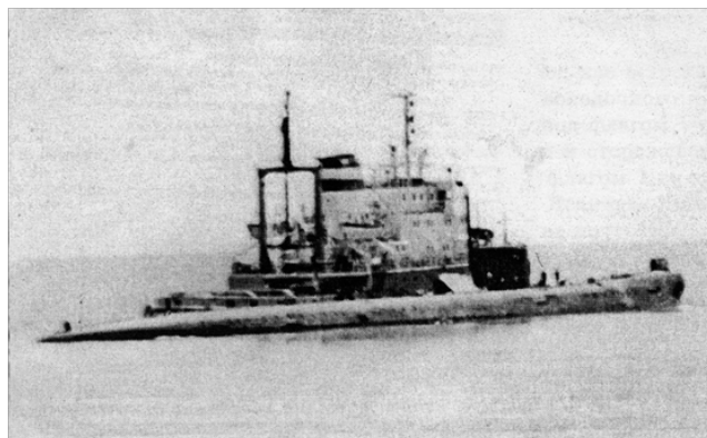
Морской буксир МБ-21 заводит буксир на аварийную К-122 (Фото из книги А. Калинин)
